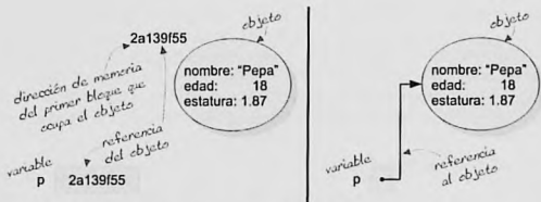
Figura 7.4. Dos formas de representar una misma referencia
