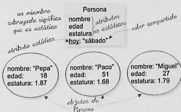
Figura 7.9. Atributo estático: hoy
