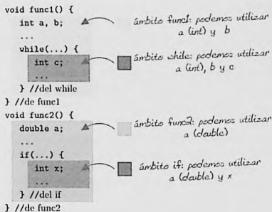
Figura 4.3. Ámbitos de distintas variables
