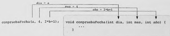
Figura 4.4. Paso de parámetros a una función
