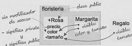
Figura 7.16. Visibilidad de private, public y por defecto
