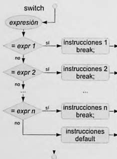
Figura 2.4. Funcionamiento de la instrucción switch con break
