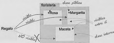
Figura 7.15. Paquete floristeria , con distinta visibilidad en sus clases
