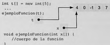
Figura 5.10. Paso de parámetro de una tabla
