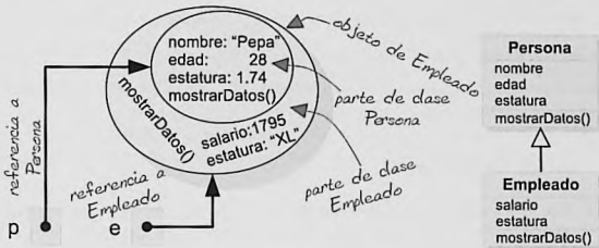
Figura 8.4. Objeto de Empleado
