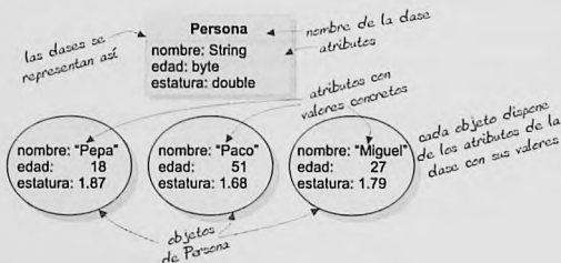
Figura 7.3. Ejemplo de valores de atributos para personas
