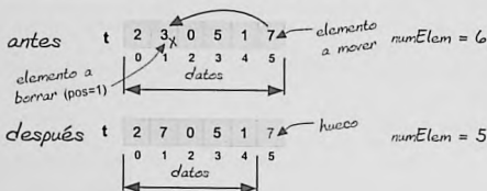
Figura 5.11. Borrado en una tabla no ordenada
