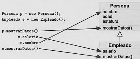
Figura 8.3. Overriding de Empleado
