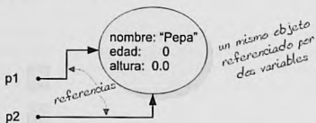
Figura 7.5. Dos formas de ver una misma referencia
