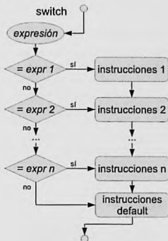
Figura 2.3. Funcionamiento de la instrucción switch
