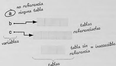
Figura 5.7. Variables y tablas
