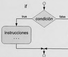
Figura 2.1. Funcionamiento de la instrucción if
