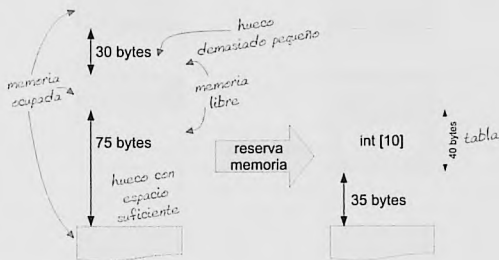
Figura 5.4. Reserva de memoria. Representación de la memoria antes y después de construir una tabla
