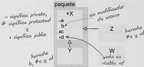
Figura 8.2. Visibilidad de un miembro protected
